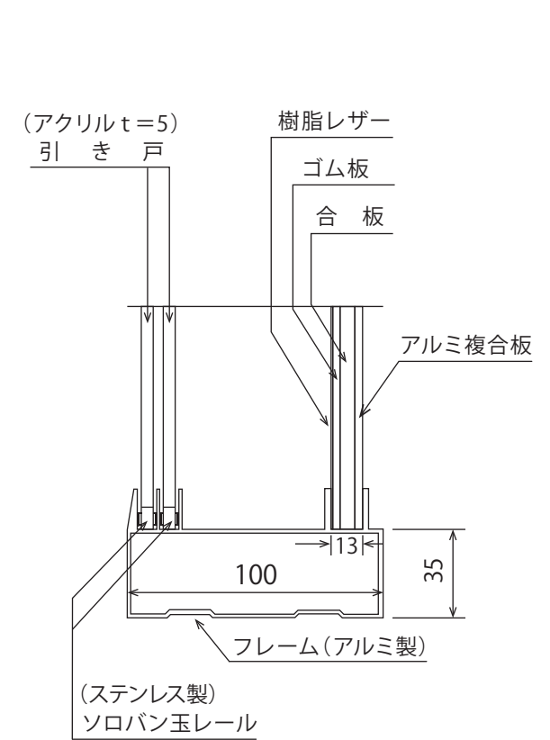
矢視 A
