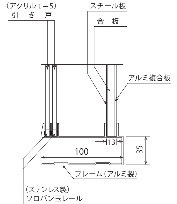
矢視 A
