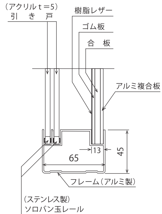
矢視 A
