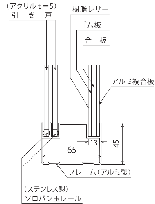
矢視 A
