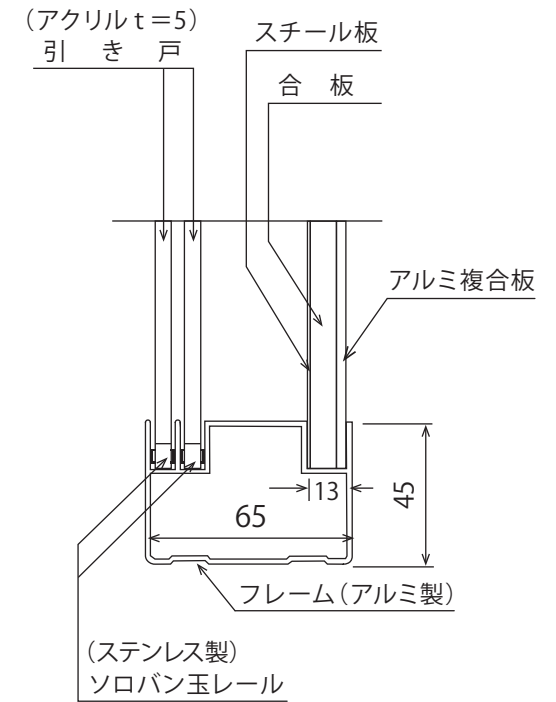
矢視 A
