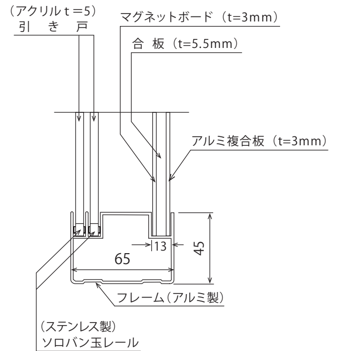
矢視 A
