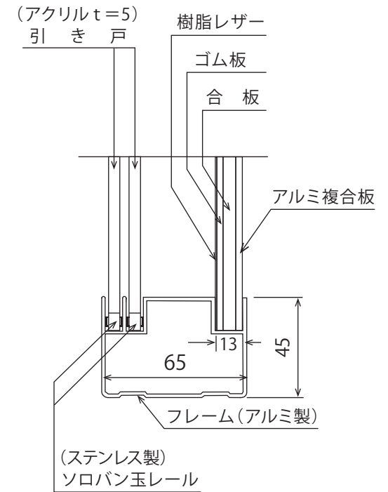
矢視 A
