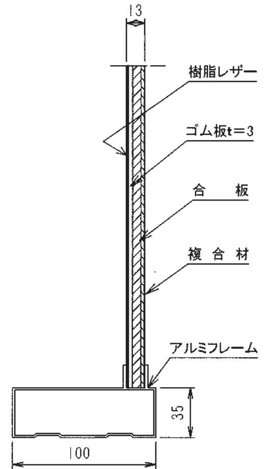
矢視A
