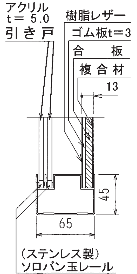
矢視 A
