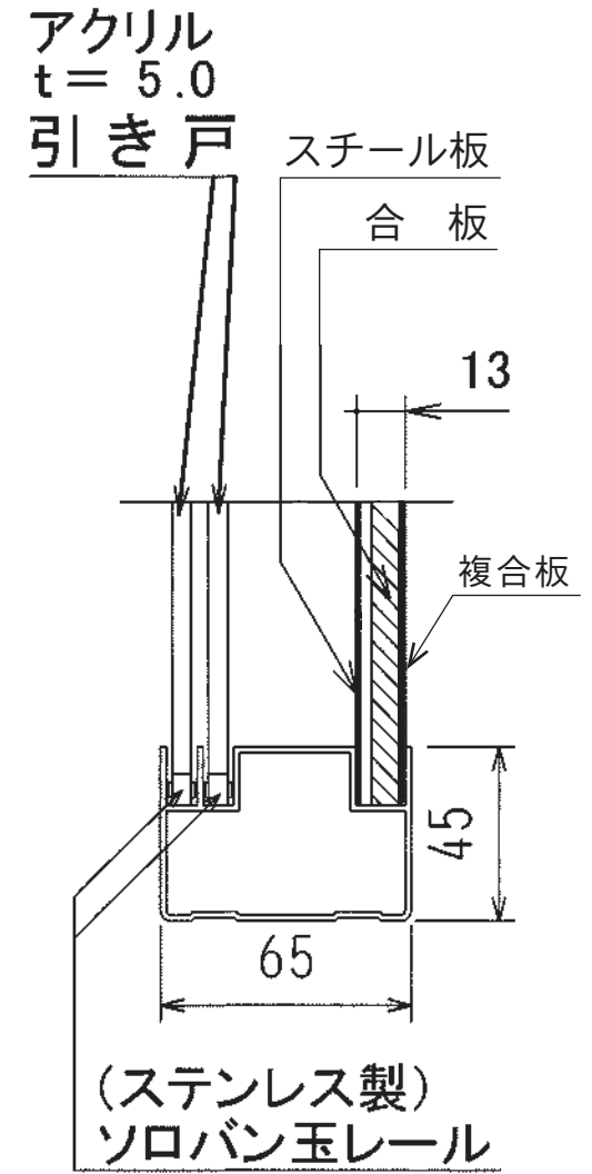
矢視 A
