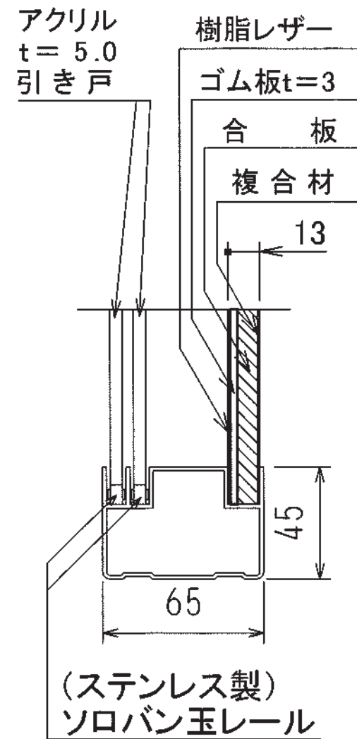
矢視 A
